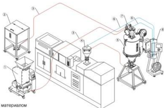
Модель 900G2 (двухступенчатый конвейер)
